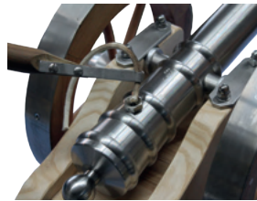
Abb. 42: Vorderladerkanone mit Luntenstockanzündung
